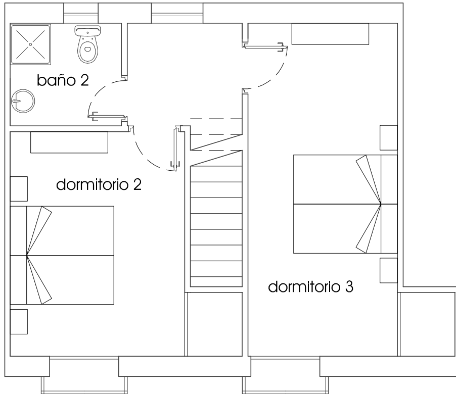
planta primera
