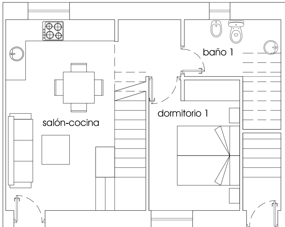
planta baja
